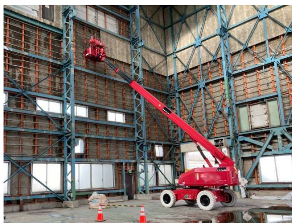
選別棟 内装解体状況
