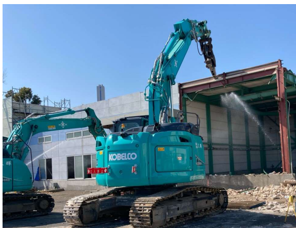
倉庫・修理棟 躯体解体状況
