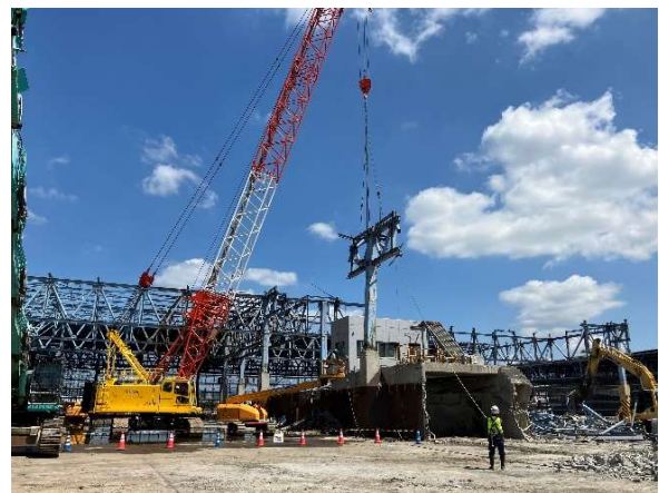
受入貯留ヤード 躯体解体状況
