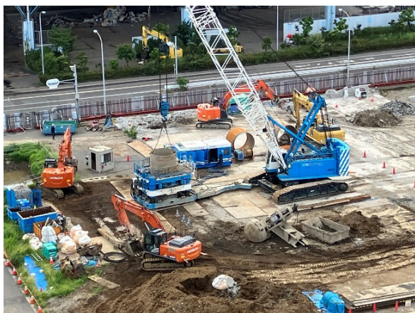
破碎機 基礎解体状況
