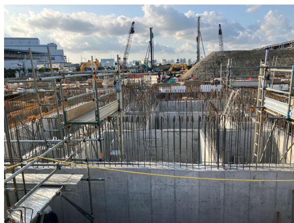
選別処理棟 汚水処理設備出来形状況
