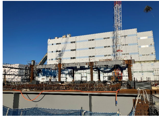
選別処理棟 鉄骨建方状況
