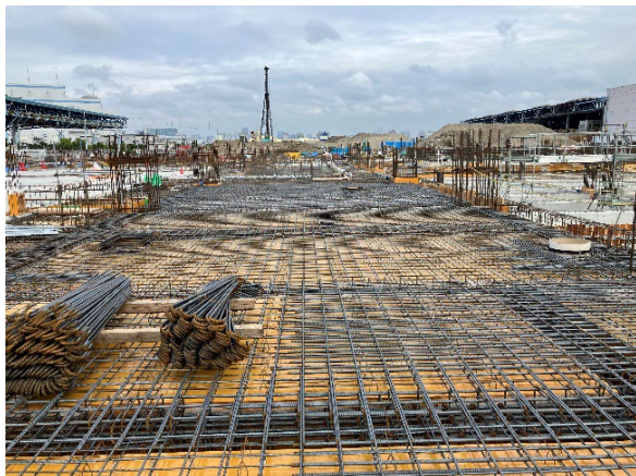
選別処理棟 スラブ配筋状況
