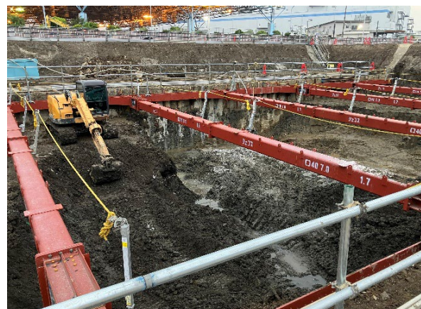
受入貯留ヤード棟 二次根伐状況
