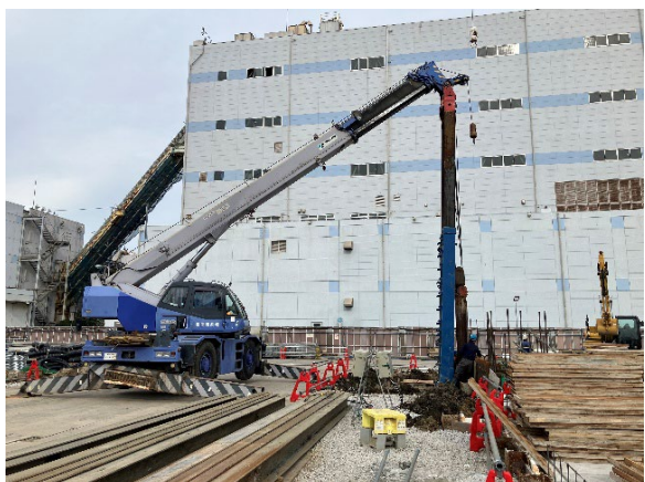
選別処理棟 山留引抜状況
