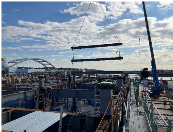
選別処理棟 鉄骨建方状況
