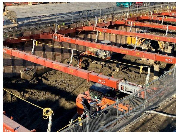
受入貯留ヤード棟 2次根伐状況
