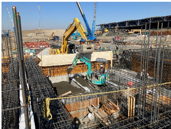
破碎処理棟 埋め戻し状況
