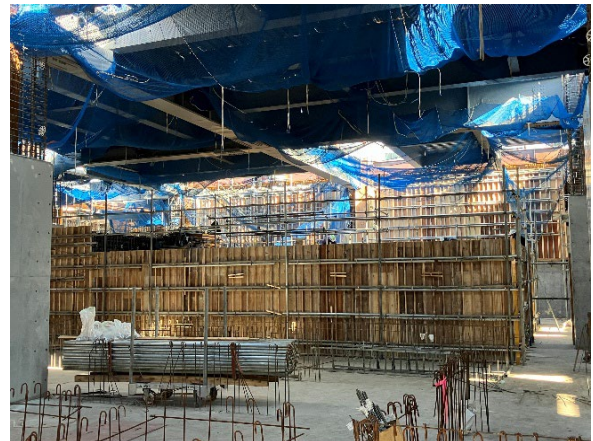
選別処理棟 汚水処理水槽型枠建込状況
