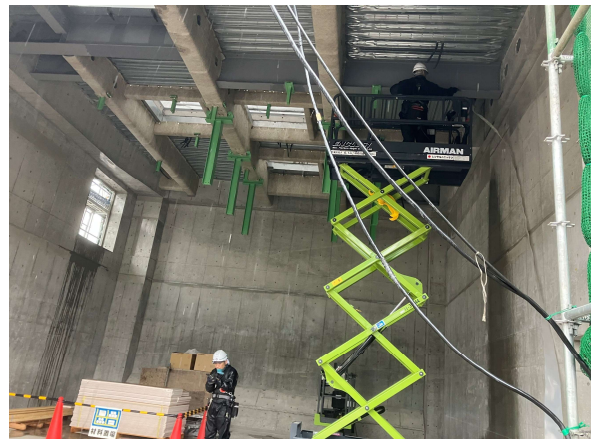
選別処理棟 耐火被覆施工状況
