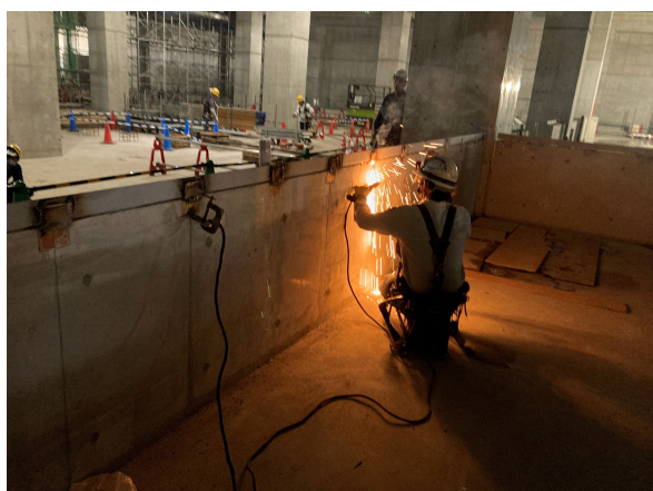
選別処理棟 1階ALC下地取付状況
